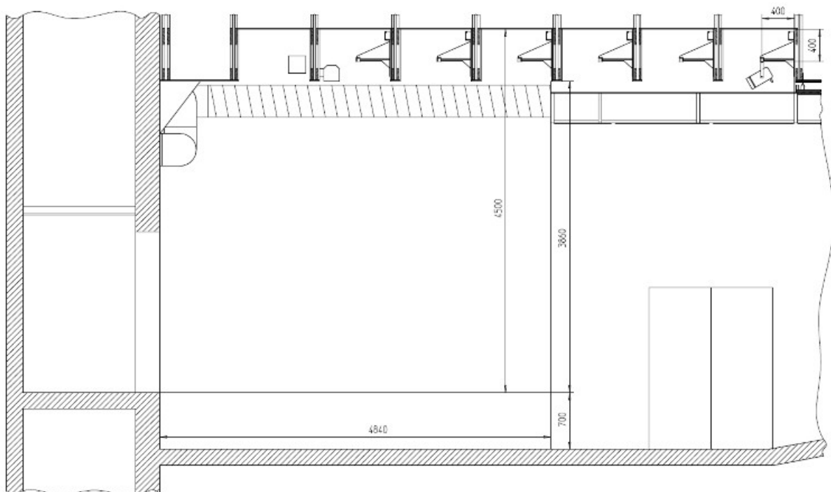
Querschnitt der Bühne mit dem rückwärtigen Abgang zum Schminkraum.
